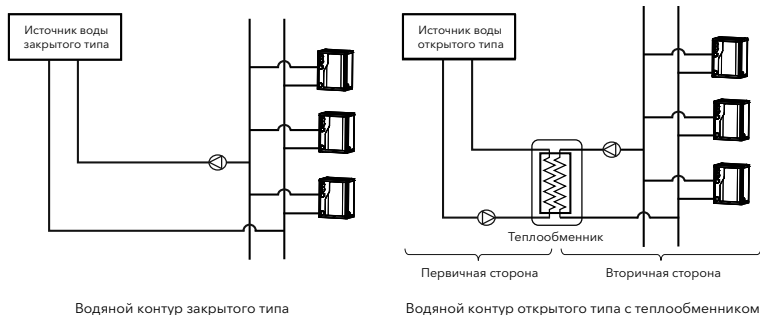
Водяной контур закрытого типа
