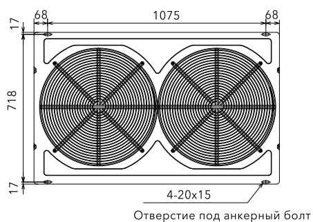
ERXY-725/800 Единица измерения: мм
