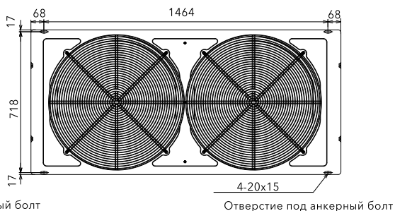
Расположение анкерных болтов
