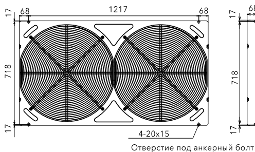
Расположение анкерных болтов
