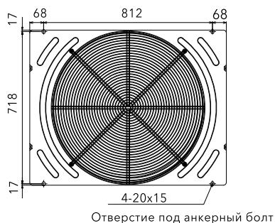
ERXY-560/615/680 Единица измерения: мм
