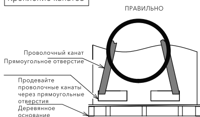
Крепление канатов
